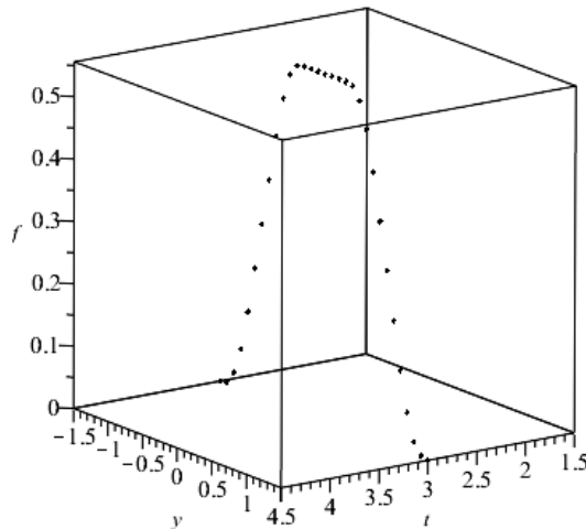
Рис. 2. Сечение f_{\eta}(y, 3)
